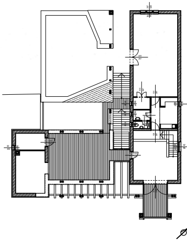
alaprajz M=1:500
