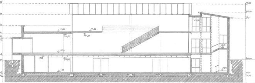
C-C VÁGAT
