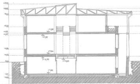
B-B VÁGAT
