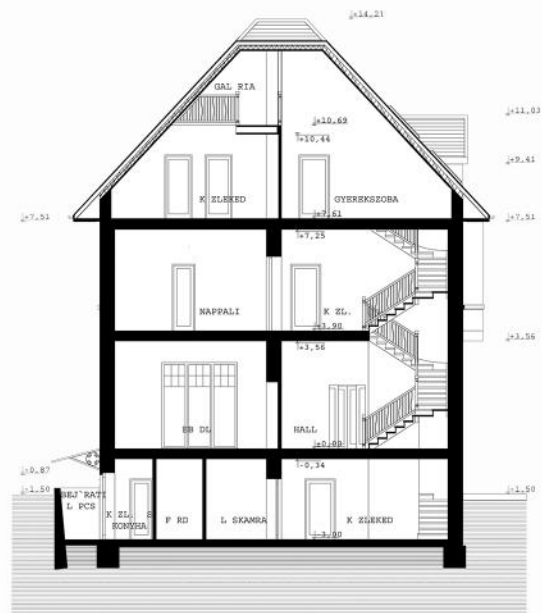
B-B KERESZTmetszet m=1:100
