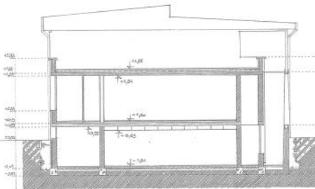
A-A VÁGAT
