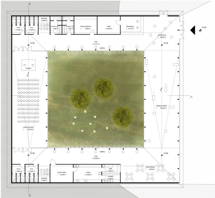
földszinti alaprajz, 1:100
