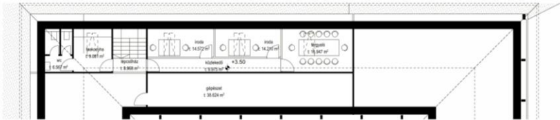
emeleti alaprajz - irodateretek, 1:100
