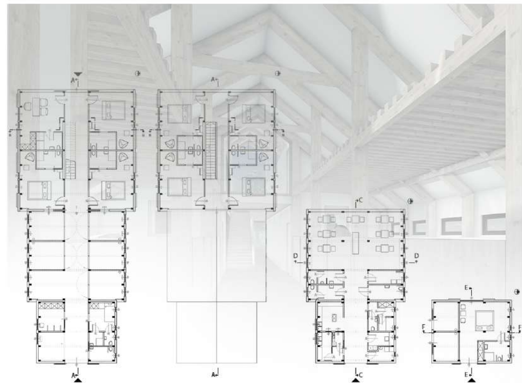
FŐÉP. FSZ. ALAPRAJZ
